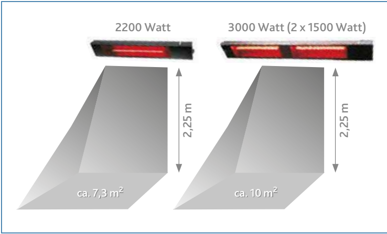
Erwärmungsflächen Infrarotheizstrahler Relax Glass io IP65
